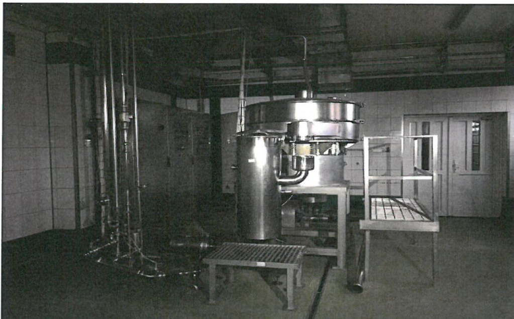
Fot.6. Widok ogólny filtra wibracyjnego. Źródło własne.
