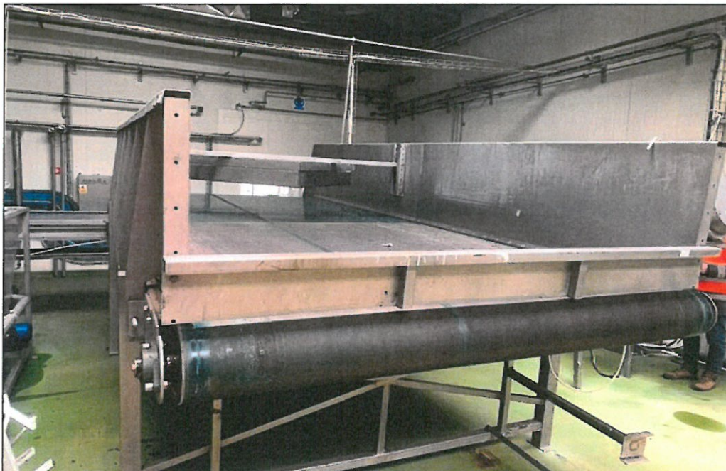
Fot.2. Widok ogólny bunkra marchwi Flottweg WM 10x4000; 2006 r. Źródło własne.
